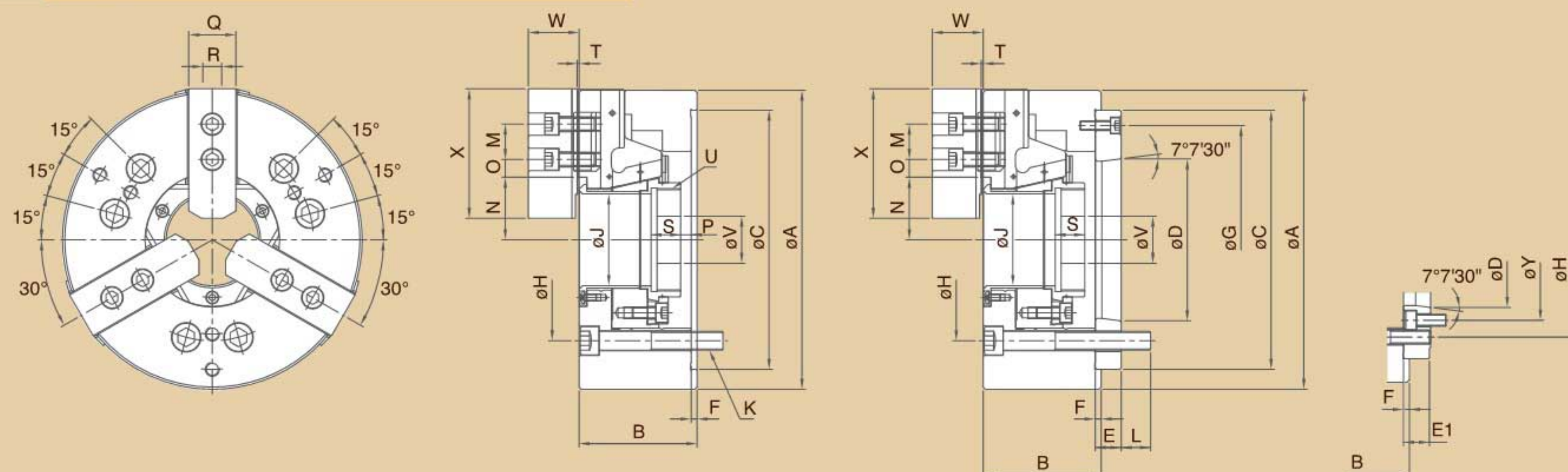
尺寸圖 » Dimensions
